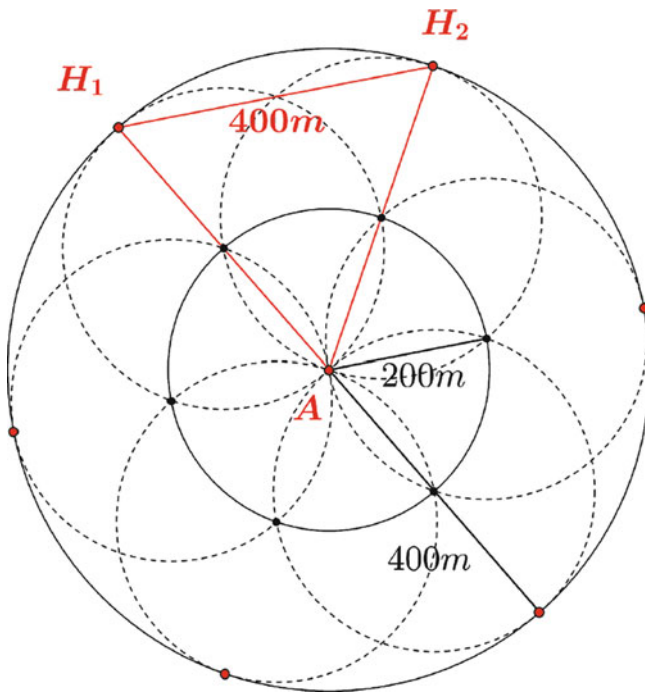
Abb. 7 Kreismodell (2) – Herleitung
