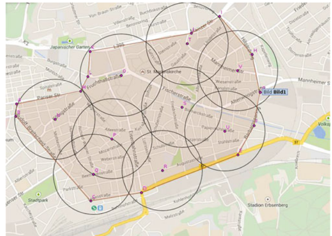
Abb. 5 Schülerlösung Kreismodell (1)
