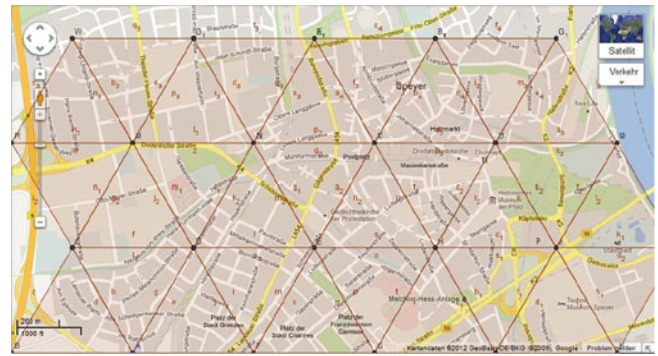
Abb. 8 Schülerlösung Dreiecksmodell
