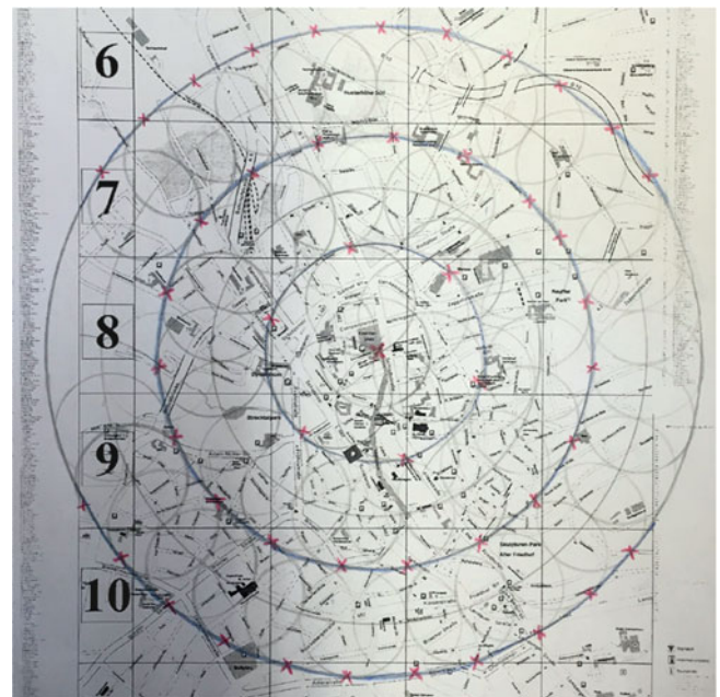
Abb. 6 Schülerlösung Kreismodell (2)
