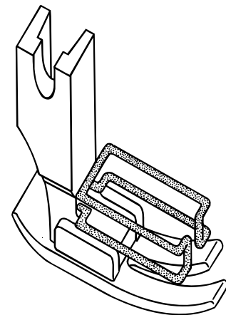
Abb. 31: Fingerabweiser
