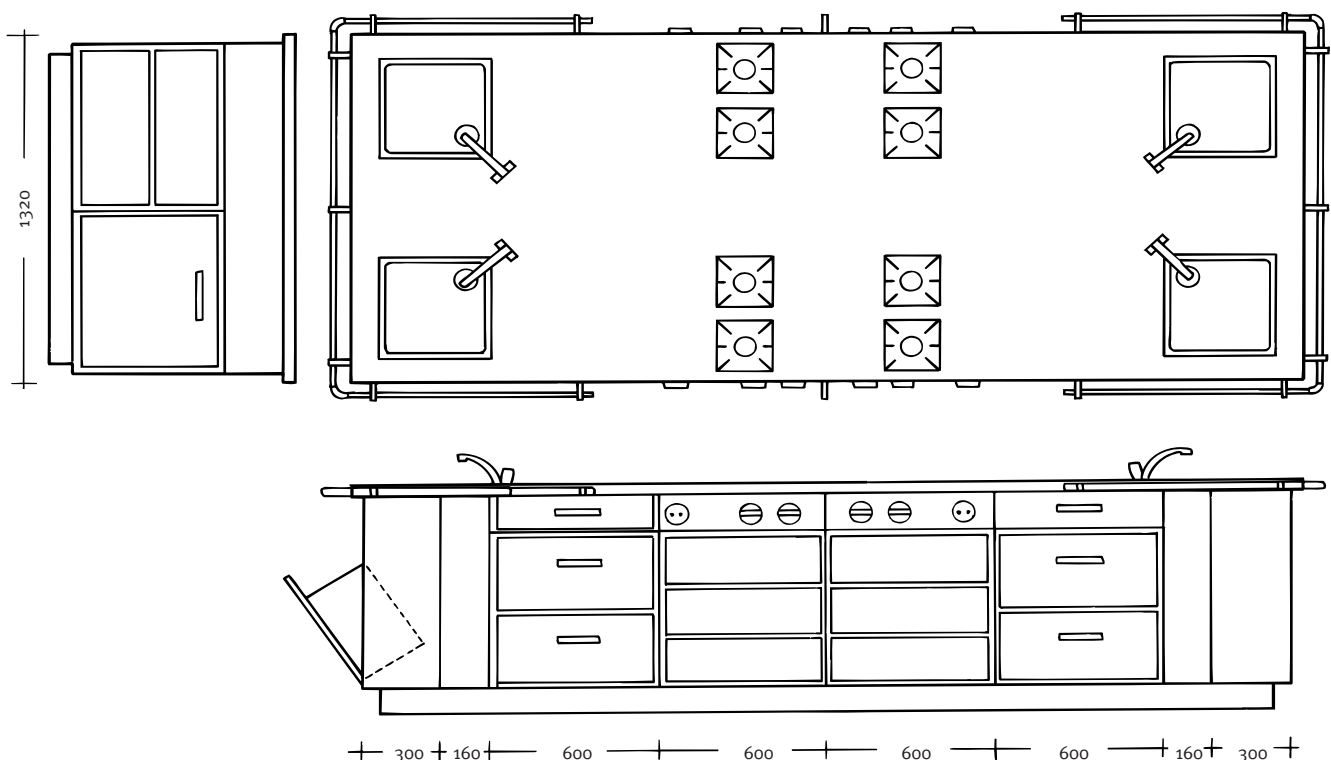
Abb. 5: Gruppeninsel
