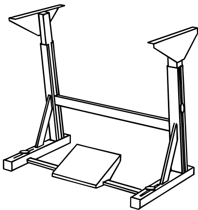
Abb. 28: Stahlprofil-Untergestell
