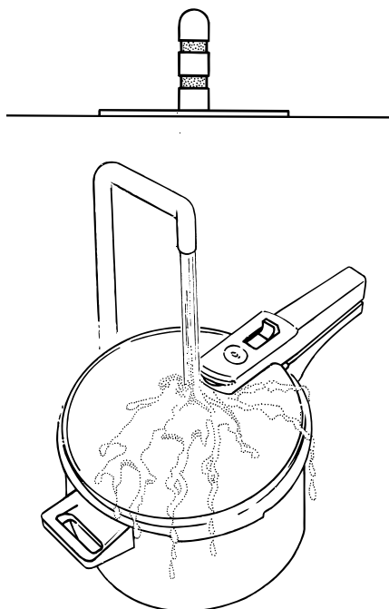
Abb. 22: Ventilstand, Abdampfen
