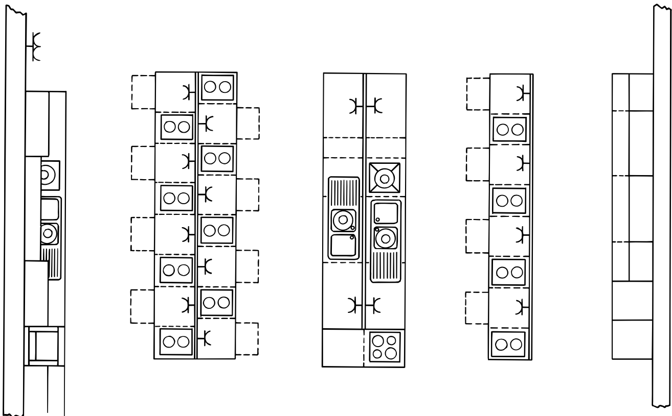
Abb. 3: Laborküche
