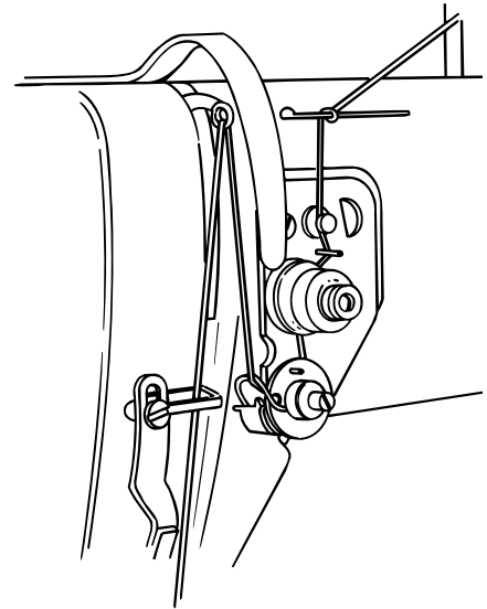
Abb. 30: Schutzbügel am Fadengeber
