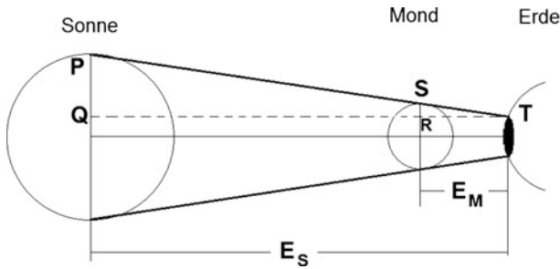
Abb. 8 Sonne–Mond–Erde, ähnliche Dreiecke
